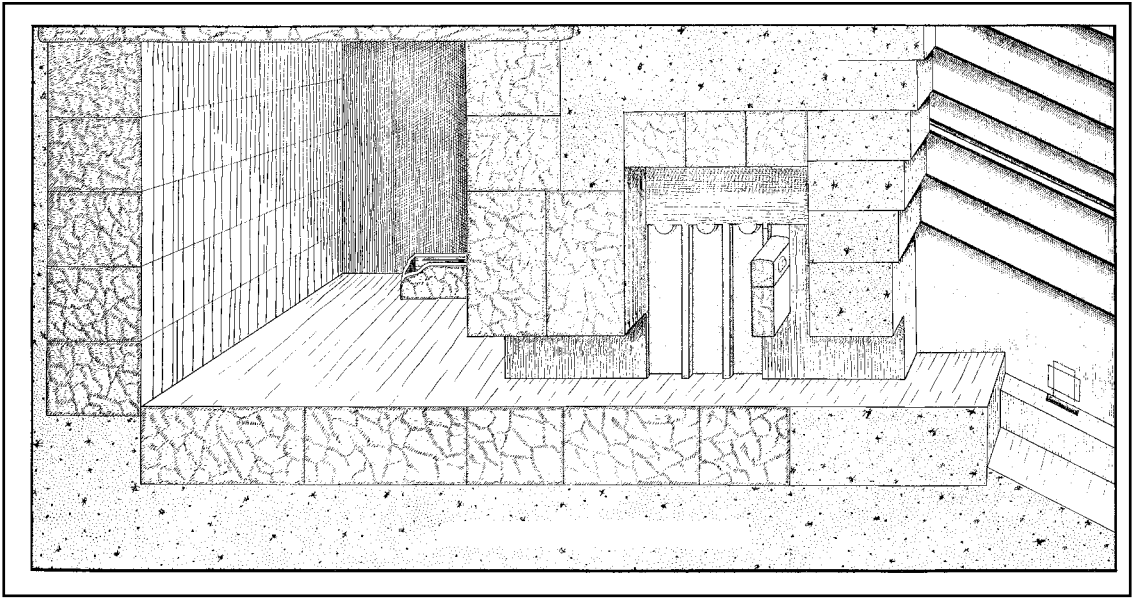
圖表 10.21 – 切面：對國王墓室及接待廳前廳的仔細觀察，顯示到處都採用了花崗岩石材和紅色花崗岩。也顯示出大階梯和大走廊的南部。圖解原作：霍華德 B. 蘭特，1933 年，蒙準使用。
