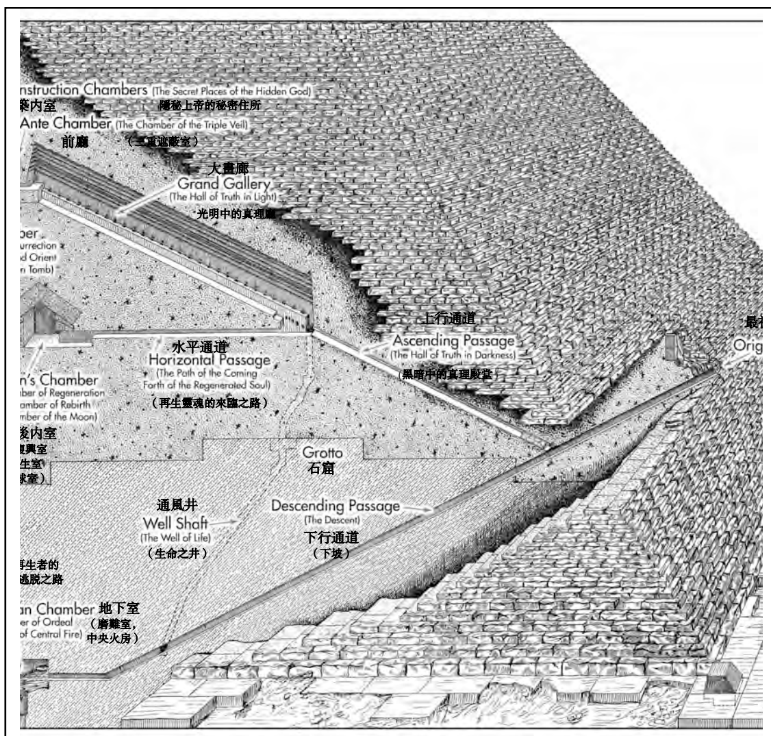
圖表 10.20 – 大金字塔的通道和內室及其名稱的切面觀察，括號內的名稱引自《埃及亡靈書》。圖解原作：霍華德 B. 蘭特，1933 年，蒙準使用。
