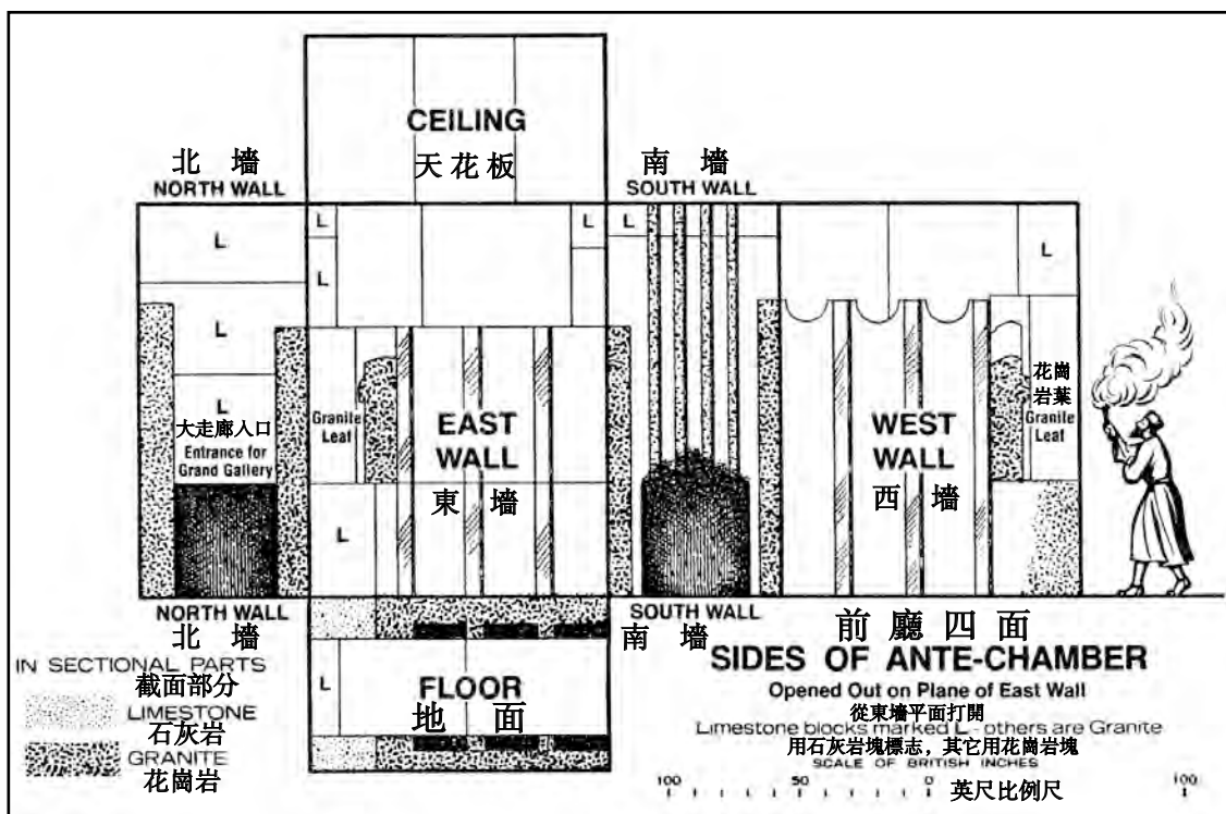
圖表 10.22 – 接待前廳四邊的詳細說明圖。
