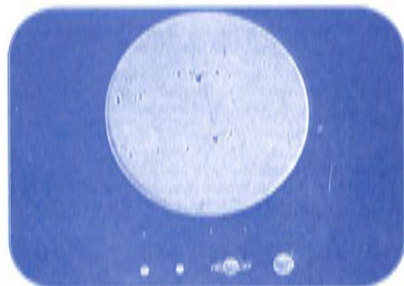
СРАВНЕНИЕ ВЕЛИКОСТИ СОЛНЦА И ПЛАНЕТ.
