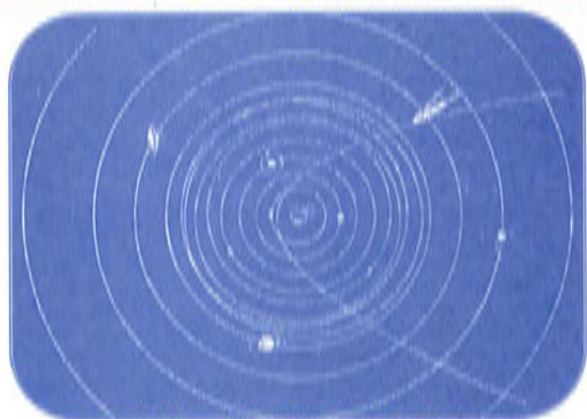
НАША ПЛАНЕТАРНАЯ СИСТЕМА.
