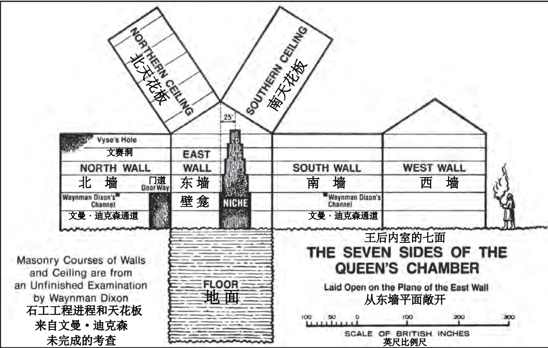
图表 10.25 - 王后墓室七面的详细说明图。
