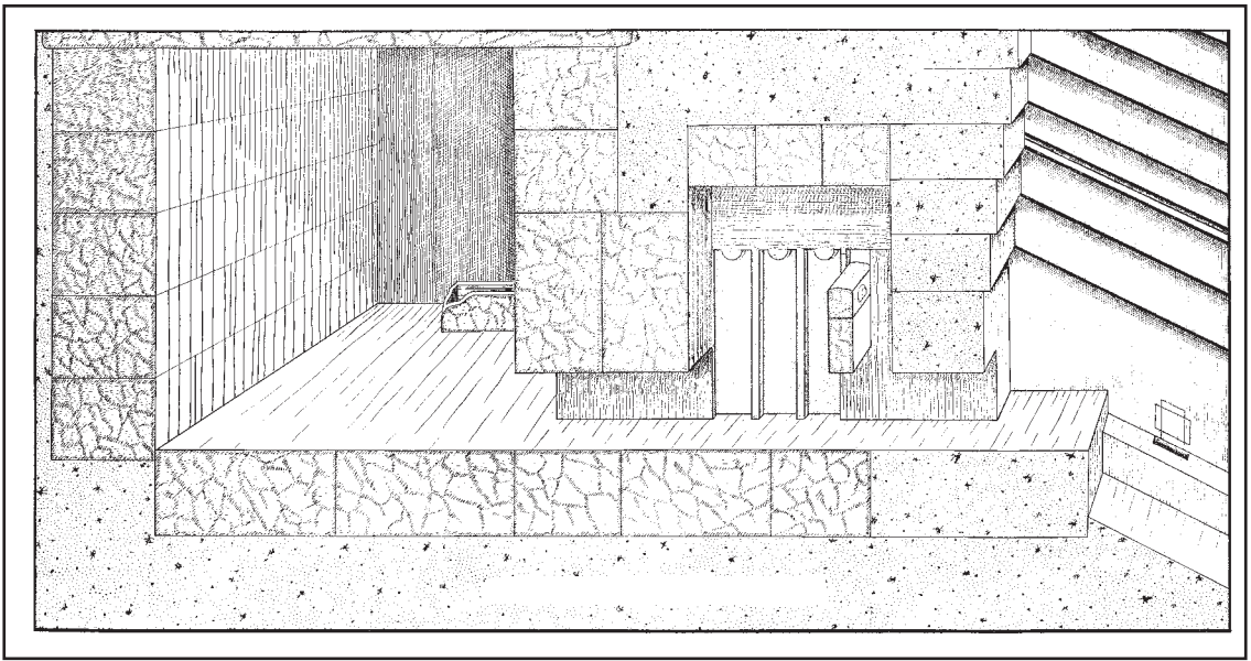
图表 10.21 - 切面：对国王墓室及接待厅前厅的仔细观察，显示到处都采用了花岗岩石材和红色花岗岩。也显示出大阶梯和大走廊的南部。图解原作：霍华德 B. 兰特，1933 年，蒙准使用。
