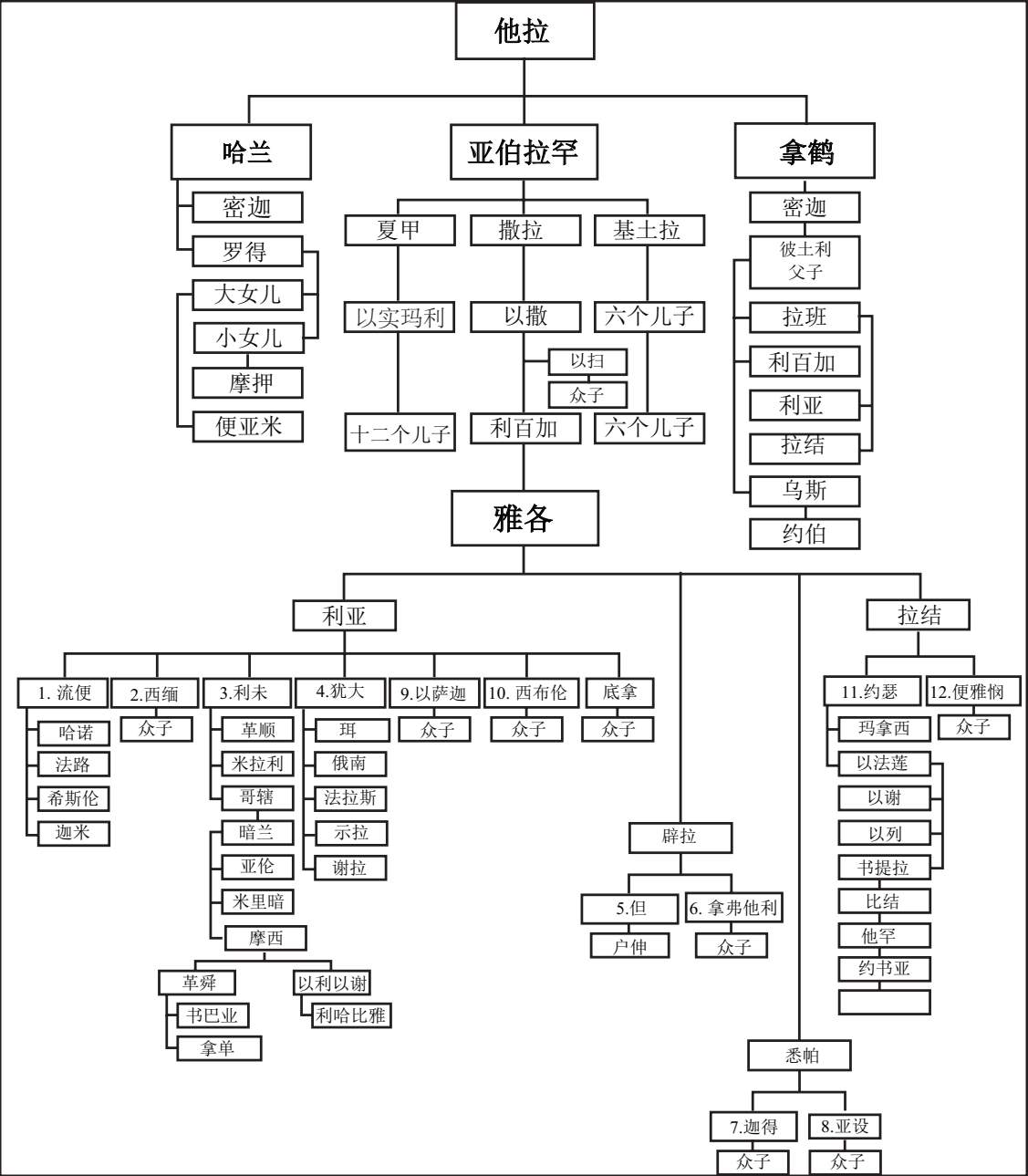
图表 8.2 - 他拉的家庭（部分）和以色列开始的宗谱图表（MS= 众子）。
