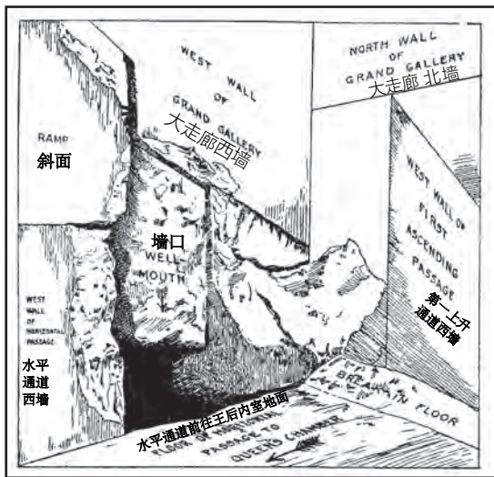
图表 10.16 - 通风井（竖井）开口通往大走廊和下降通道。
